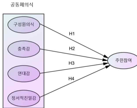
[그림 1] 연구모형
